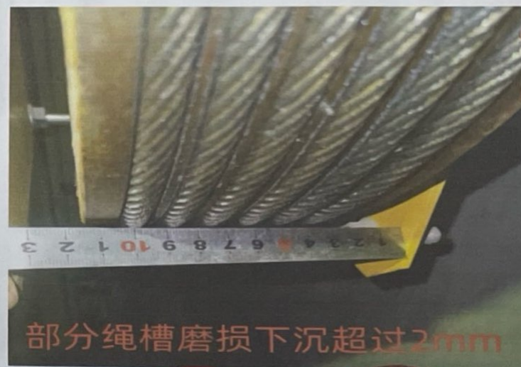
对重反绳轮
